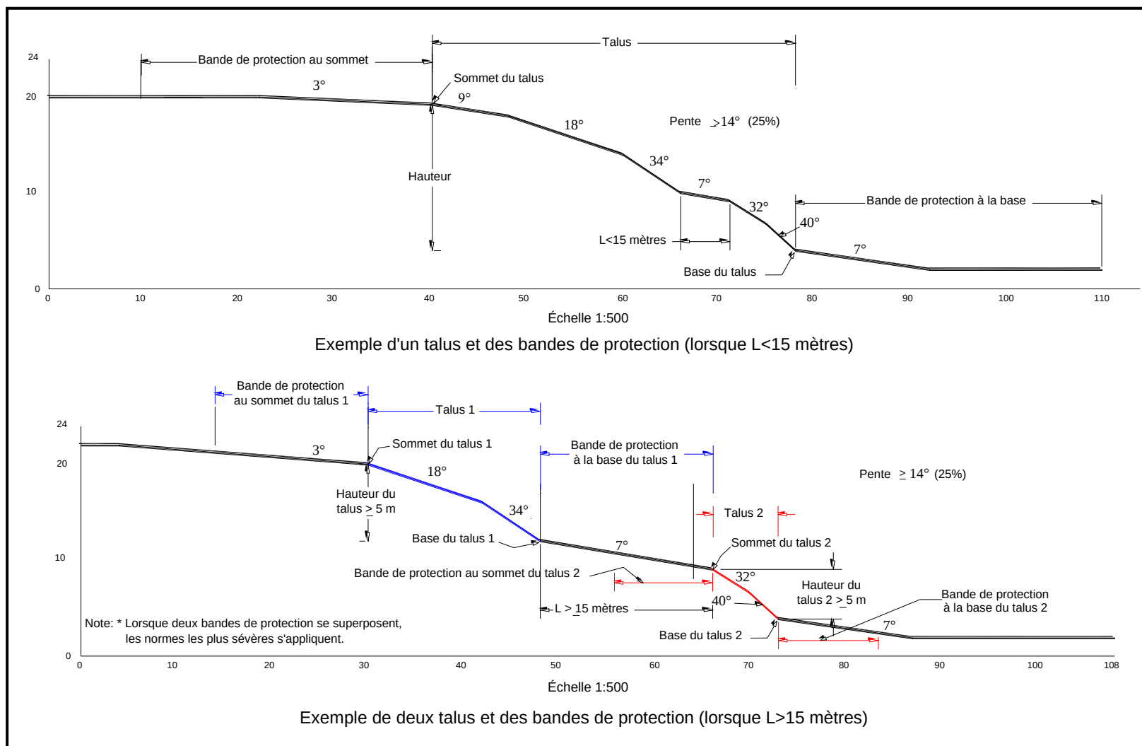
Figure 4 : Croquis d'un talus composé de sols à prédominance argileuse avec un plateau de moins de 15 m (croquis supérieur) et d'un de plus de 15 m (croquis inférieur) R-228, art. 3
